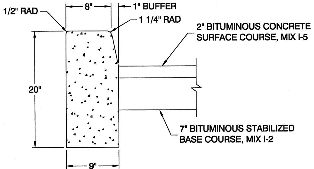
TYP 9" x 20" CURB DETAIL
